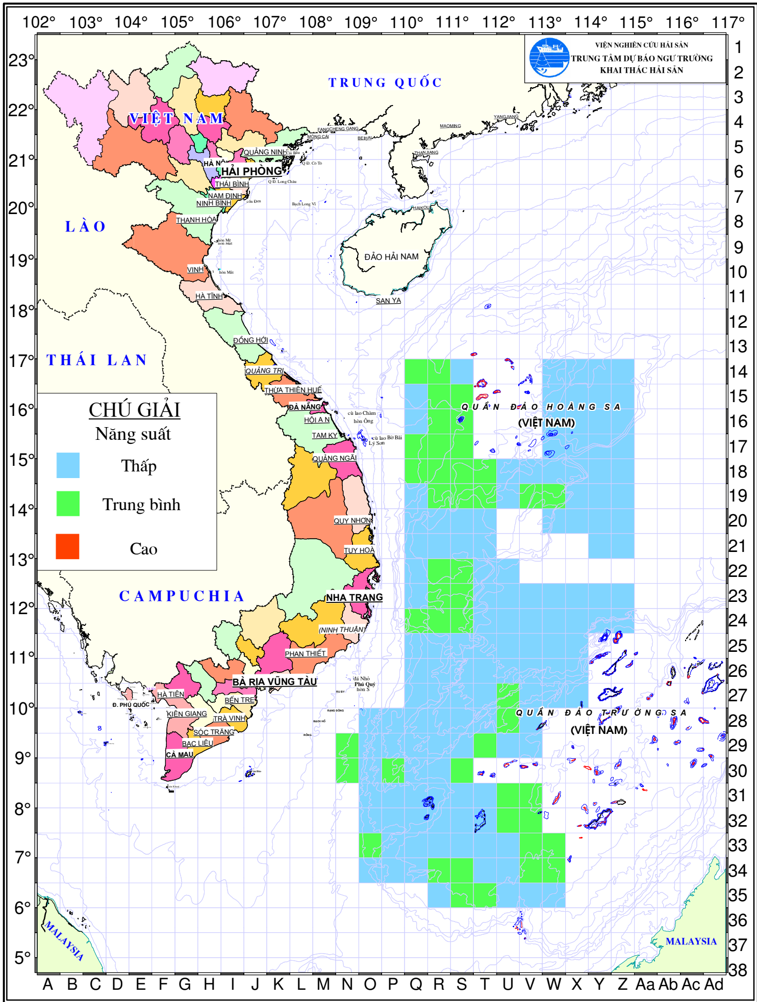
BẢN DỰ BÁO NGƯ TRƯỜNG KHAI THÁC CÁ NGỪ ĐẠI DƯƠNG TỪ NGÀY 08 ĐẾN 15 THÁNG 07 NĂM 2018
