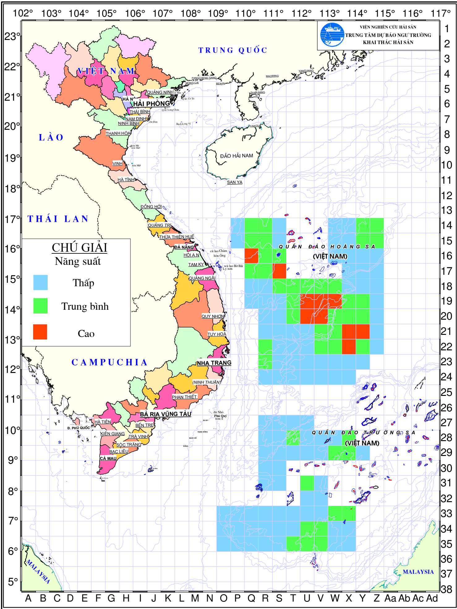
BẢN DỰ BÁO NGƯ TRƯỜNG KHAI THÁC CÁ NGỪ ĐẠI DƯƠNG TỪ NGÀY 16 ĐẾN 23 THÁNG 09 NĂM 2017
